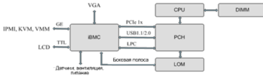
Рис. 2-1 Архитектура системы
